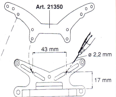
Schema di montaggio supporto posteriore per ammortizzatori a grande volume. Large volume shock-absorber mounting support.
